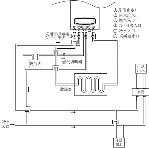
图 3 标准配管图
