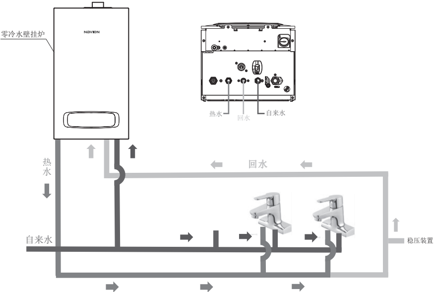
有回水管(三管式)运行原理图
