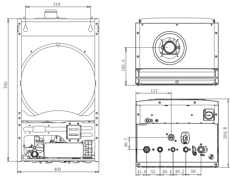
图 1 壁挂炉尺寸图
