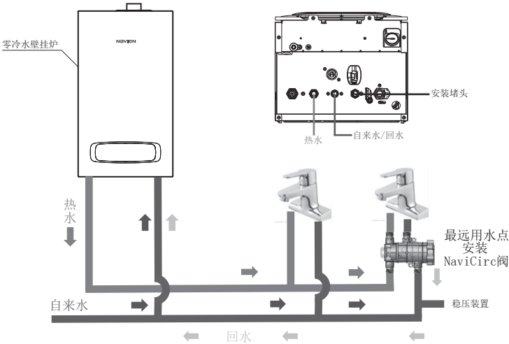
无回水管(两管式)运行原理图
