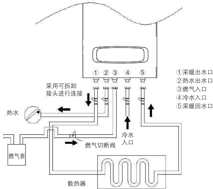
图 3 标准配管图
